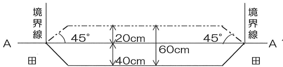
縦横断面図
