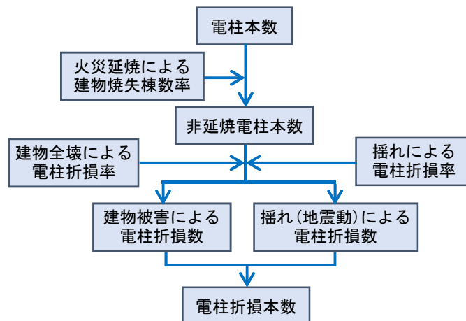
図Ⅲ. 3. 1-1 電力施設の電柱折損本数の算定フロー (中央防災会議（2013、首都直下）より抜粋)
