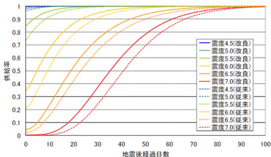
図Ⅲ.3.2-2 上水道の計測震度に対する供給率曲線の予測（能島ら(2012)※）
