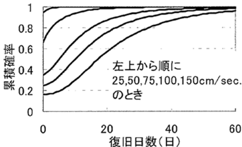
図Ⅲ. 3. 3-2 下水道の供給率復旧曲線（日下ほか，2011）
