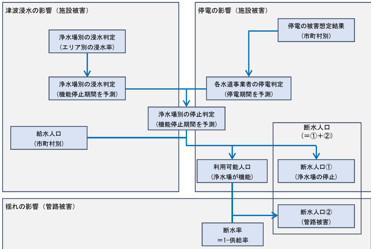
図Ⅲ.3.2-1 断水人口の算定フロー（中央防災会議（2013、首都直下）を一部修正）
