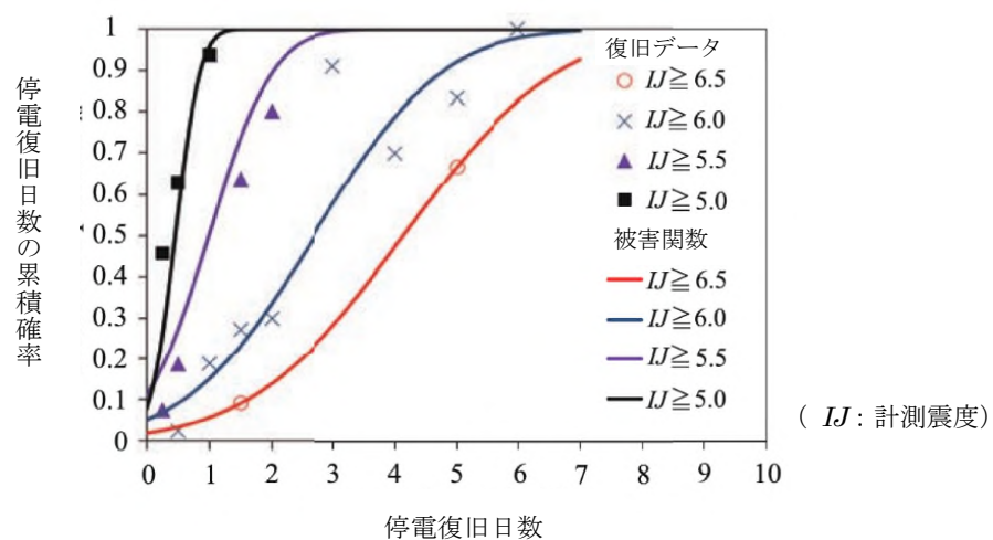
図Ⅲ.3.1-3 電力の計測震度に対する停電復旧時間の曲線 (Shoji ほか (2011))
