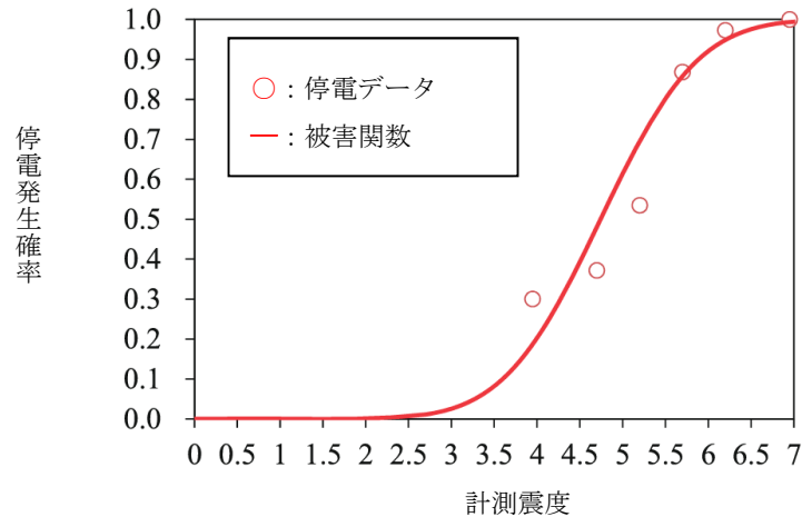
図Ⅲ.3.1-2 計測震度に対する停電発生確率 (Shoji ほか (2011))
