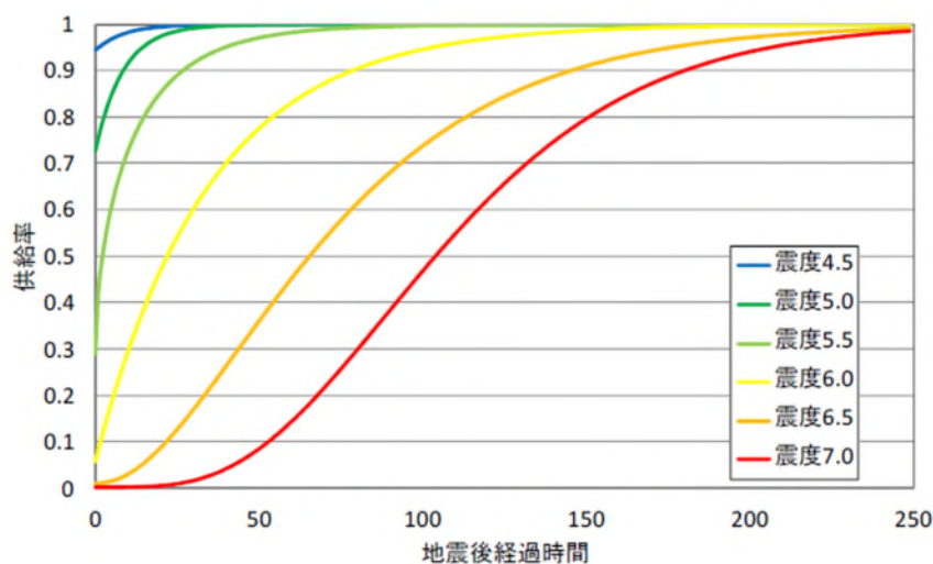
図Ⅲ. 4. 1-2 通信施設の復旧予測に活用する電力の供給率曲線
