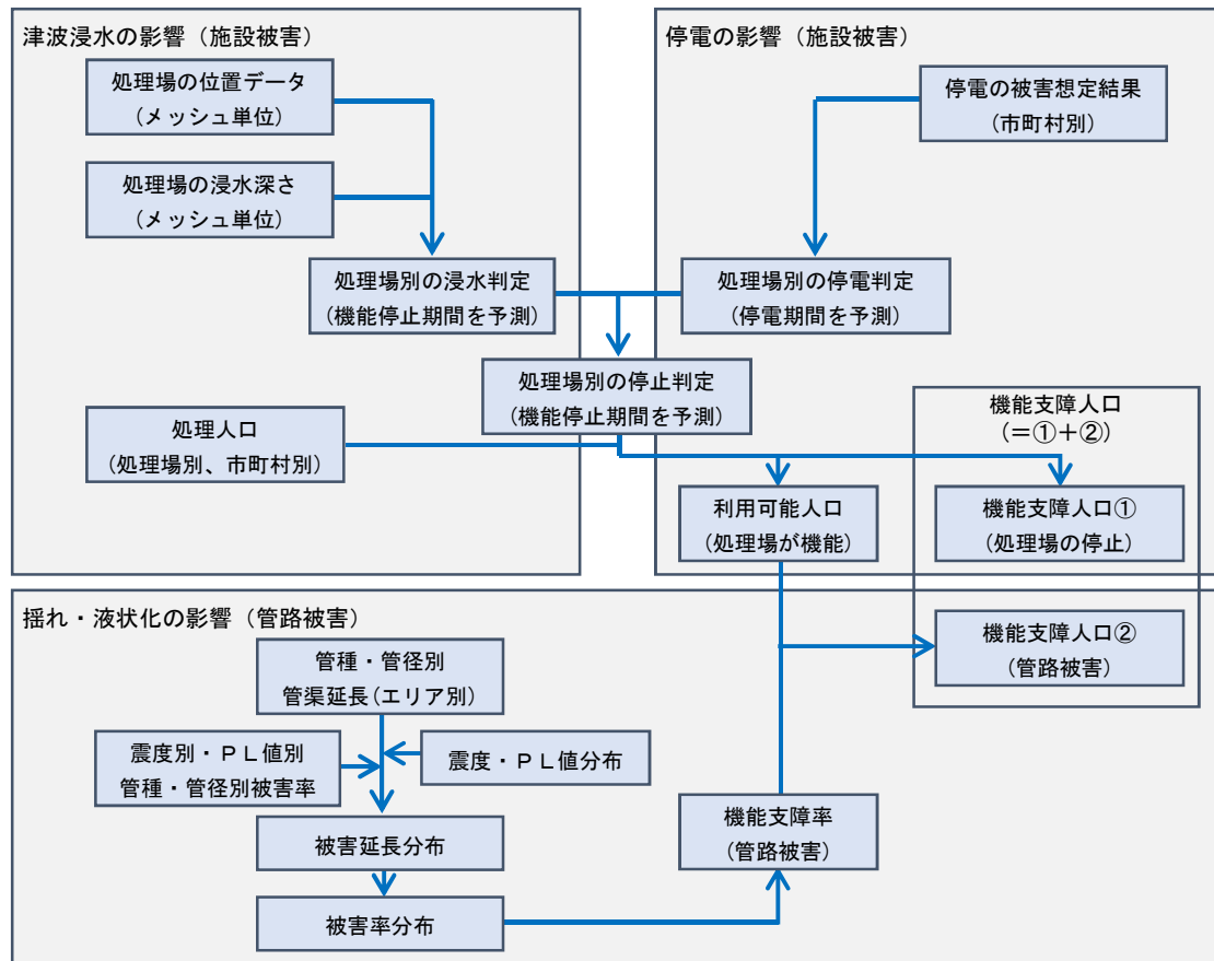
図Ⅲ.3.3-1 下水道施設の機能支障人口の算定フロー（内閣府（2013、首都直下）を一部修正）
