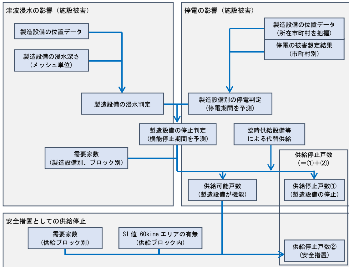
図Ⅲ.3.4-1 都市ガスの供給停止戸数の算定フロー（中央防災会議（2013、首都直下））
