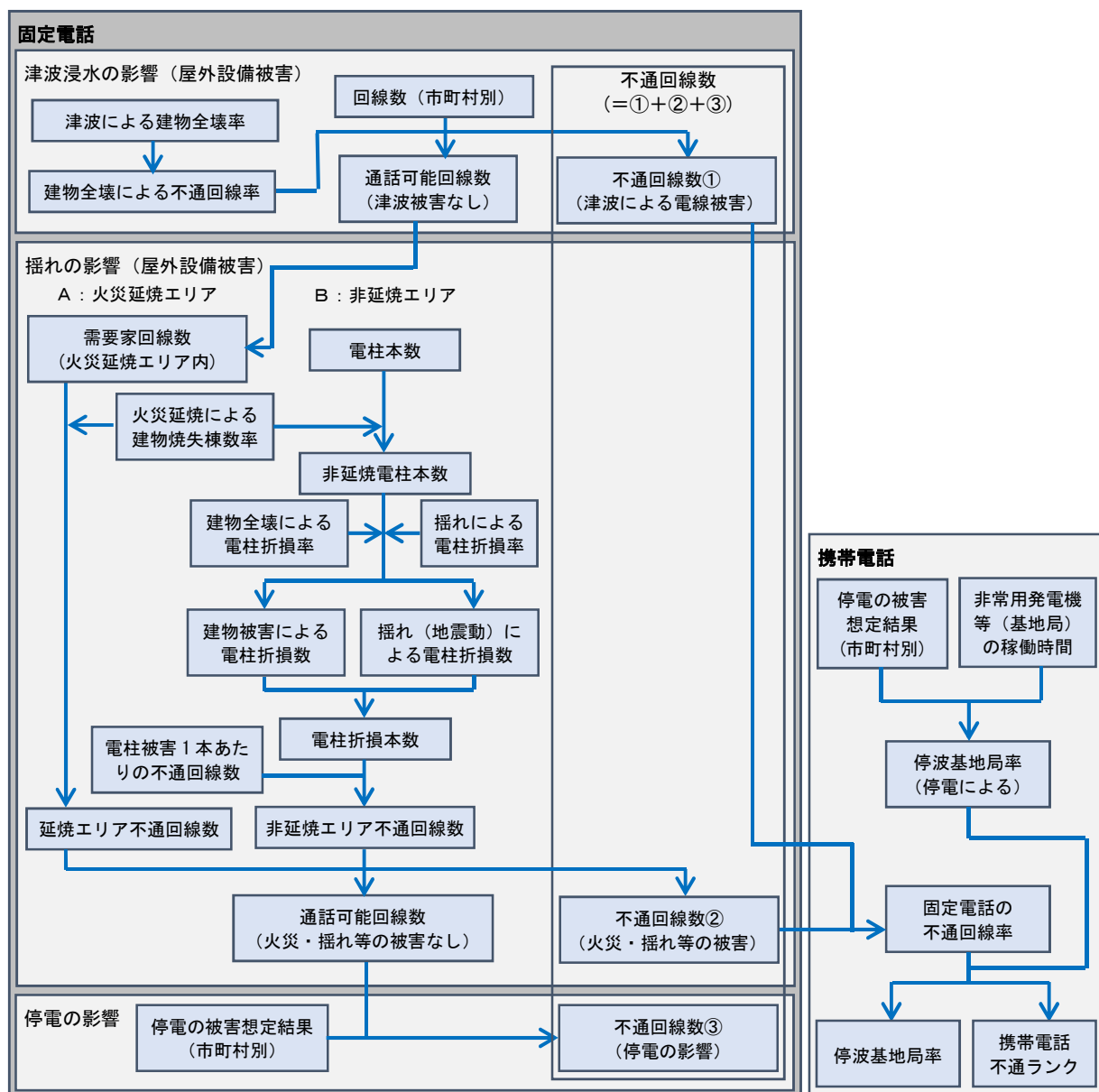
図Ⅲ.4.1-1 不通回線数、携帯電話不通ランクの算定フロー
